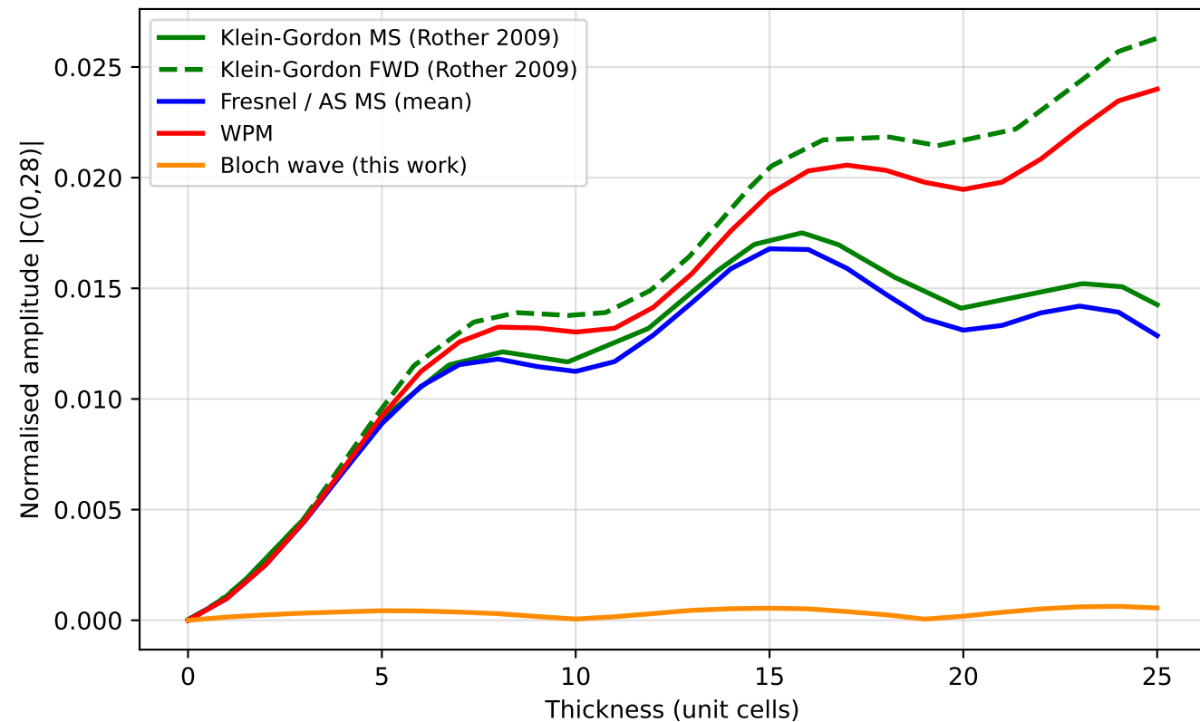
[0, 28] beam ( \approx 135 \text{ mrad} ) — Au, 300 keV
