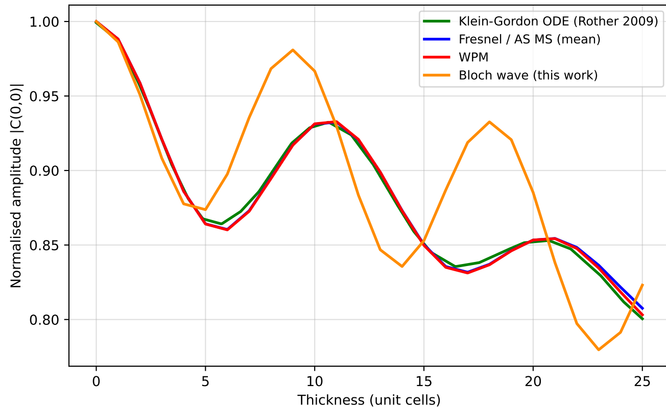
[0, 0] beam — Au, 300 keV
