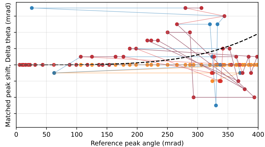
target 1270 A, actual 1272.9 A, F-MS/WPM peaks = 49
