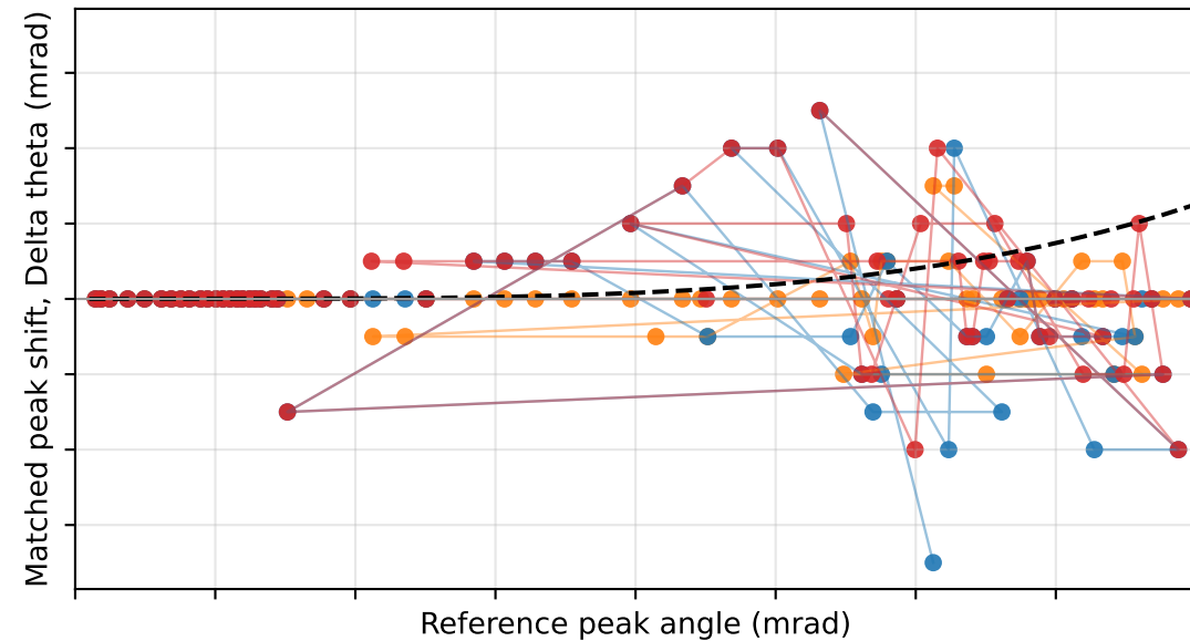
target 1270 A, actual 1272.9 A, F-MS/WPM peaks = 49
