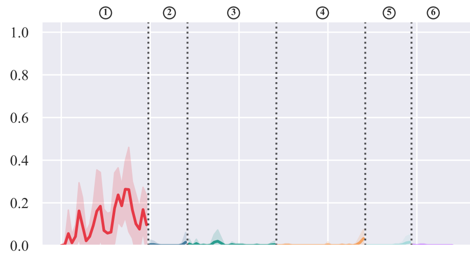
Clip Fraction
