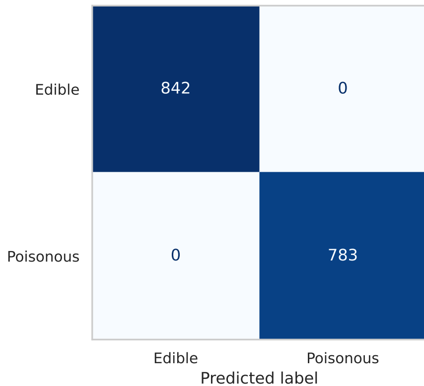
AdaBoost
