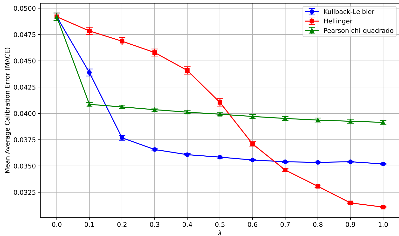
MovieLens com ALS
