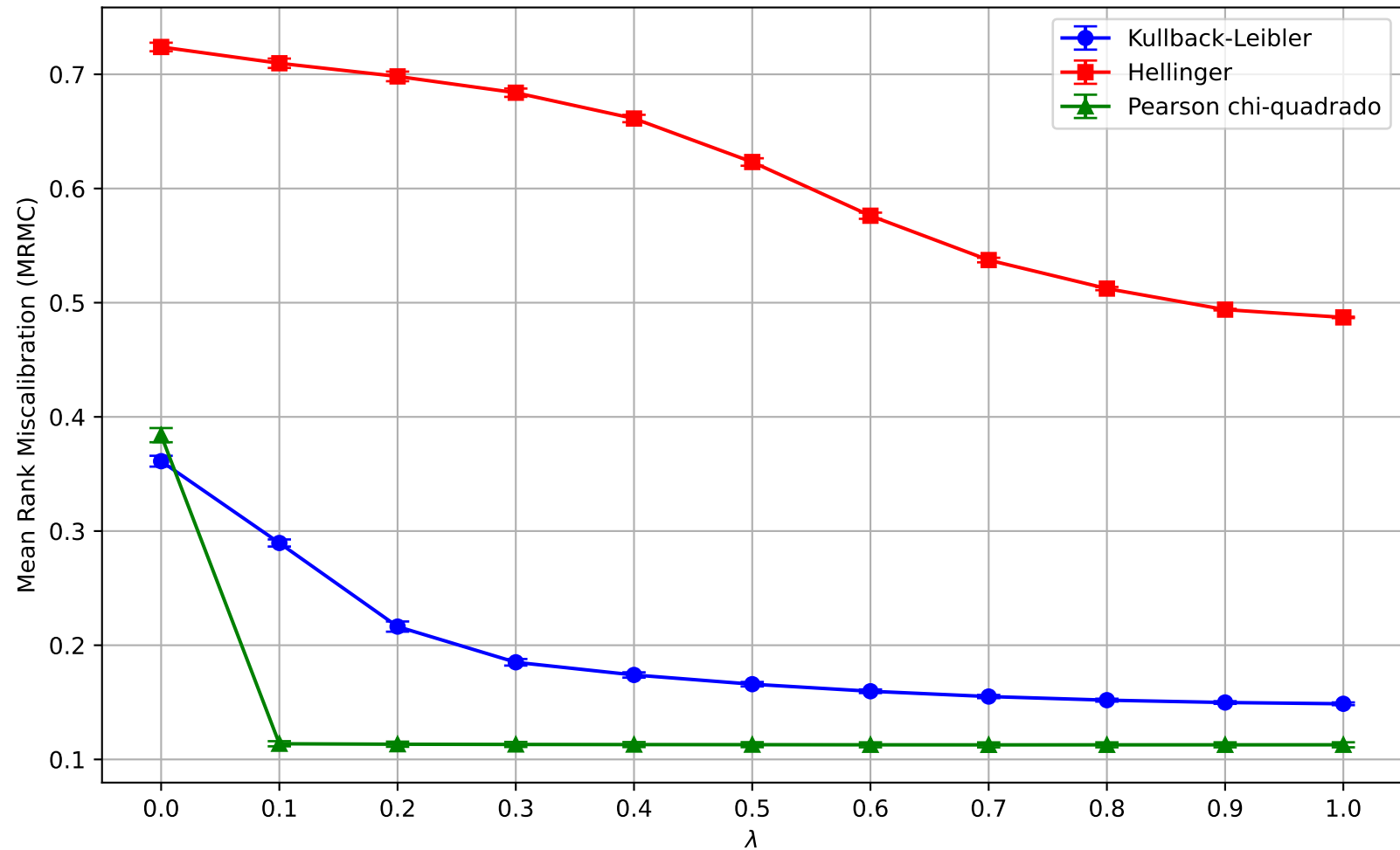
MovieLens com ALS
