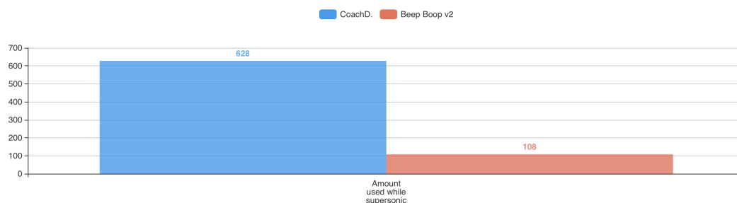
FIGURE 5 – Consommation du boost lorsque la vitesse supersonique est atteinte
