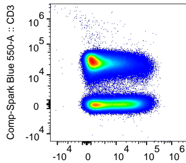
Comp-BUV563-A :: CD69
