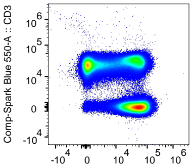
Comp-BV605-A :: CD45RA
