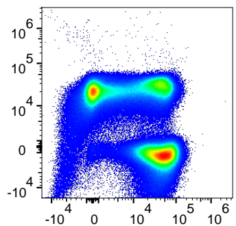
Comp-BV605-A :: CD45RA
