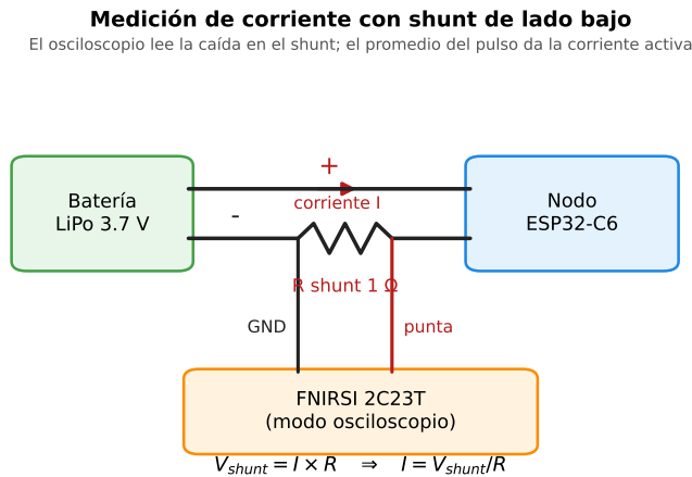
Figura 6.1: Montaje documentado para medir corriente a partir de la caída en un shunt de lado bajo. Explica la conexión y conversión tensión–corriente; no acredita una captura experimental del pulso ni la corriente total de sueño. Fuente: diagrama del repositorio.
