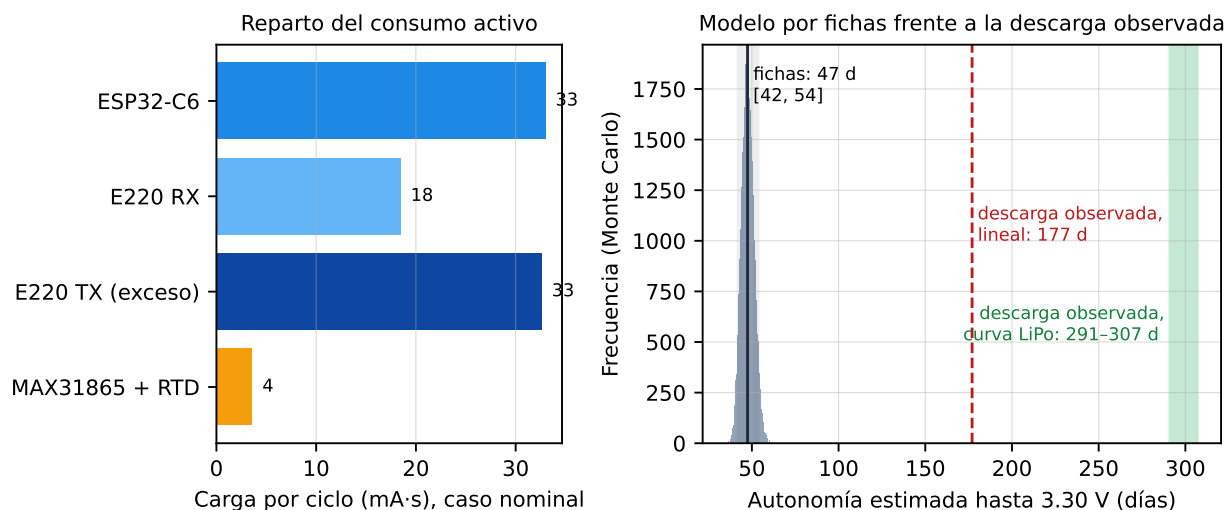
Figura 9.9: Modelo de consumo por estados con valores de ficha: reparto de la carga por ciclo en el caso nominal y distribución Monte Carlo de la autonomía, frente a las dos proyecciones de la descarga observada. Fuente: analisis/modelo_consumo.py.
