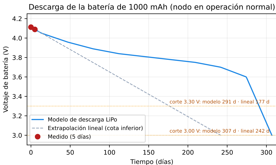
Figura 9.8: Descarga parcial de cinco días con la celda de 1000 mAh: los dos puntos de tensión medidos y las dos extrapolaciones, lineal y por curva típica LiPo. La curva lineal, rotulada en la figura como cota conservadora, es el menor de los dos modelos; ninguna de las dos es una descarga completa medida de la celda. Fuente: figura de analisis/autonomia_bateria.py.
