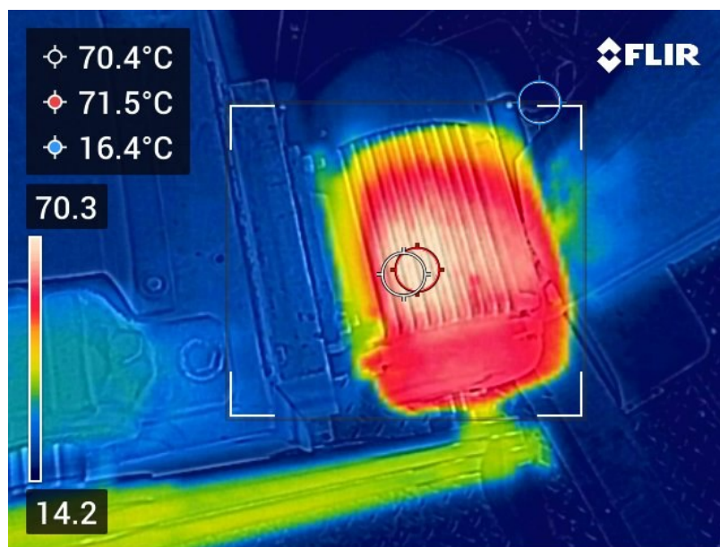
Figura 9.11: Imagen térmica del motor del succionador, tomada según el registro de campo con una cámara FLIR C8, que localiza el punto caliente sobre la carcasa. Sirve como contexto espacial del calentamiento; no identifica su causa mecánica. Fuente: evidencia fotográfica del proyecto.
