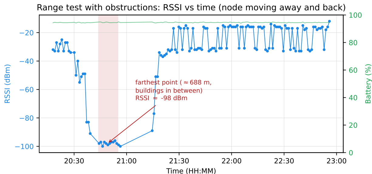
Figura 9.7: RSSI y porcentaje indicado de batería durante el recorrido móvil con obstrucciones. El enlace seguía operativo cerca de 688 m; la abscisa es tiempo, no distancia fija controlada. Fuente: figura existente de analisis/prueba_distancia.py.
