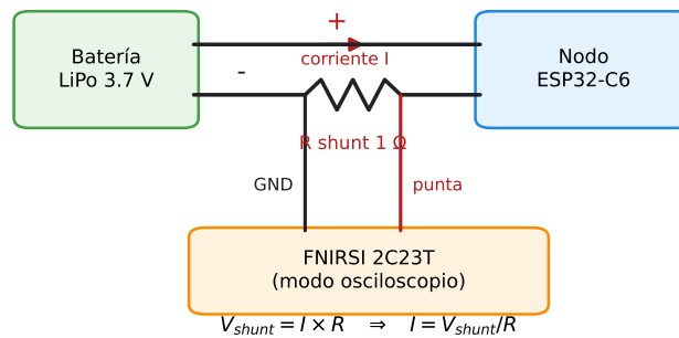
Figura 6.1: Montaje para medir la corriente del nodo con un shunt de lado bajo y un osciloscopio; la caída de tensión en el shunt se convierte en corriente. Es el esquema propuesto: el pulso activo y la corriente de sueño no llegaron a registrarse. Fuente: diagrama del repositorio.
