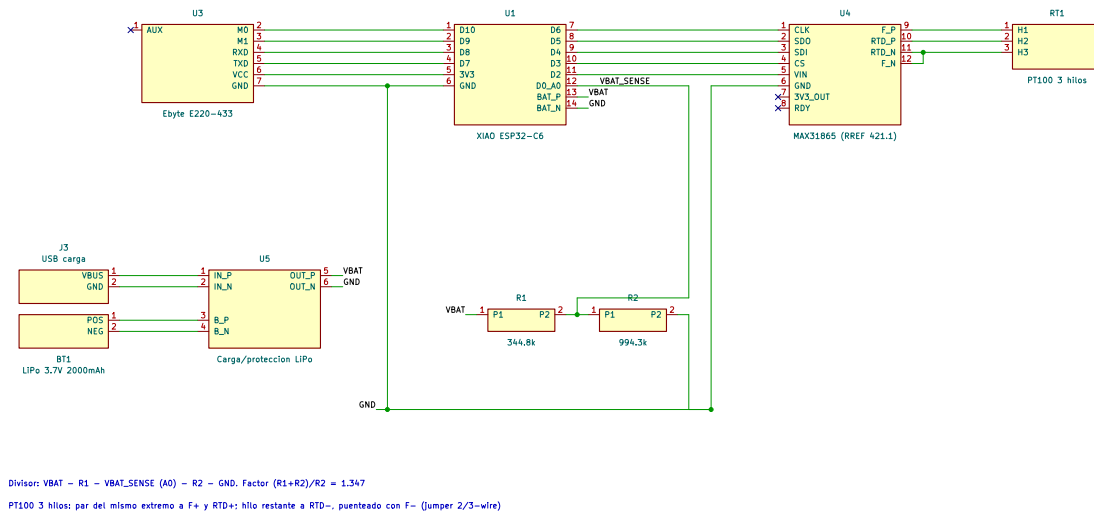
Figura 8.2: Conexiones del nodo: SPI hacia el MAX31865, UART y líneas de modo hacia el E220, alimentación y divisor de batería. Los rótulos identifican el tipo de componente, no la referencia comercial exacta de la sonda ni del radio. Fuente: esquema del proyecto.
