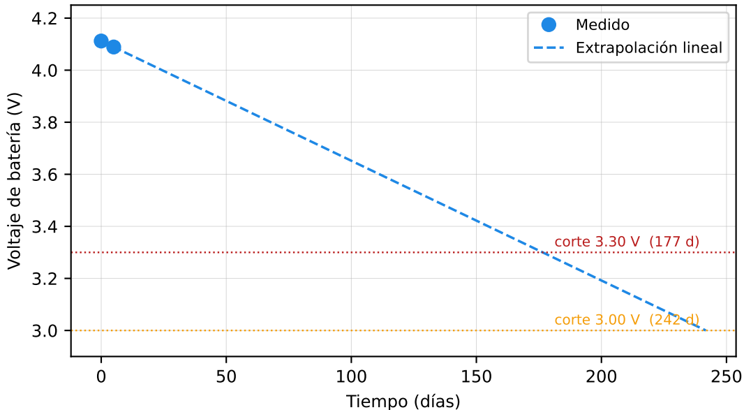
Descarga de la batería de 1000 mAh (nodo en operación normal)
