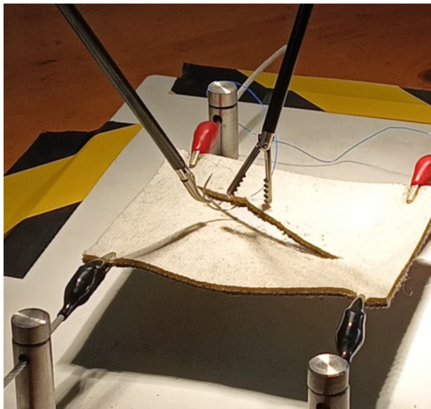
FIGURA 4.22: Prueba de sutura sobre el kit de entrenamiento de cirugía laparoscópica
