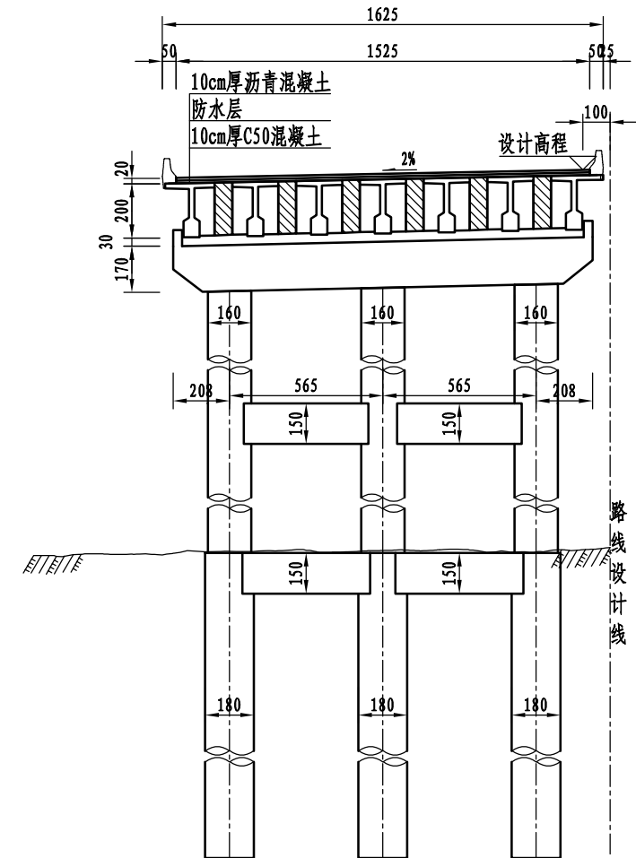
III-III 左半幅
