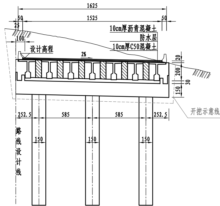
I-I 左半幅
