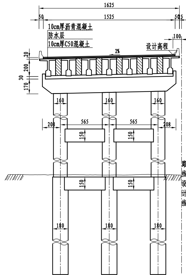
II-II 左半幅
