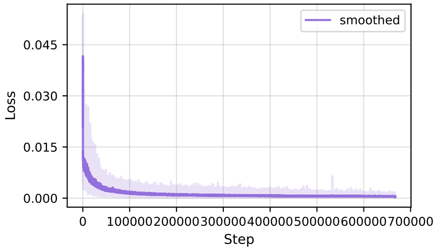
SSI MSE
