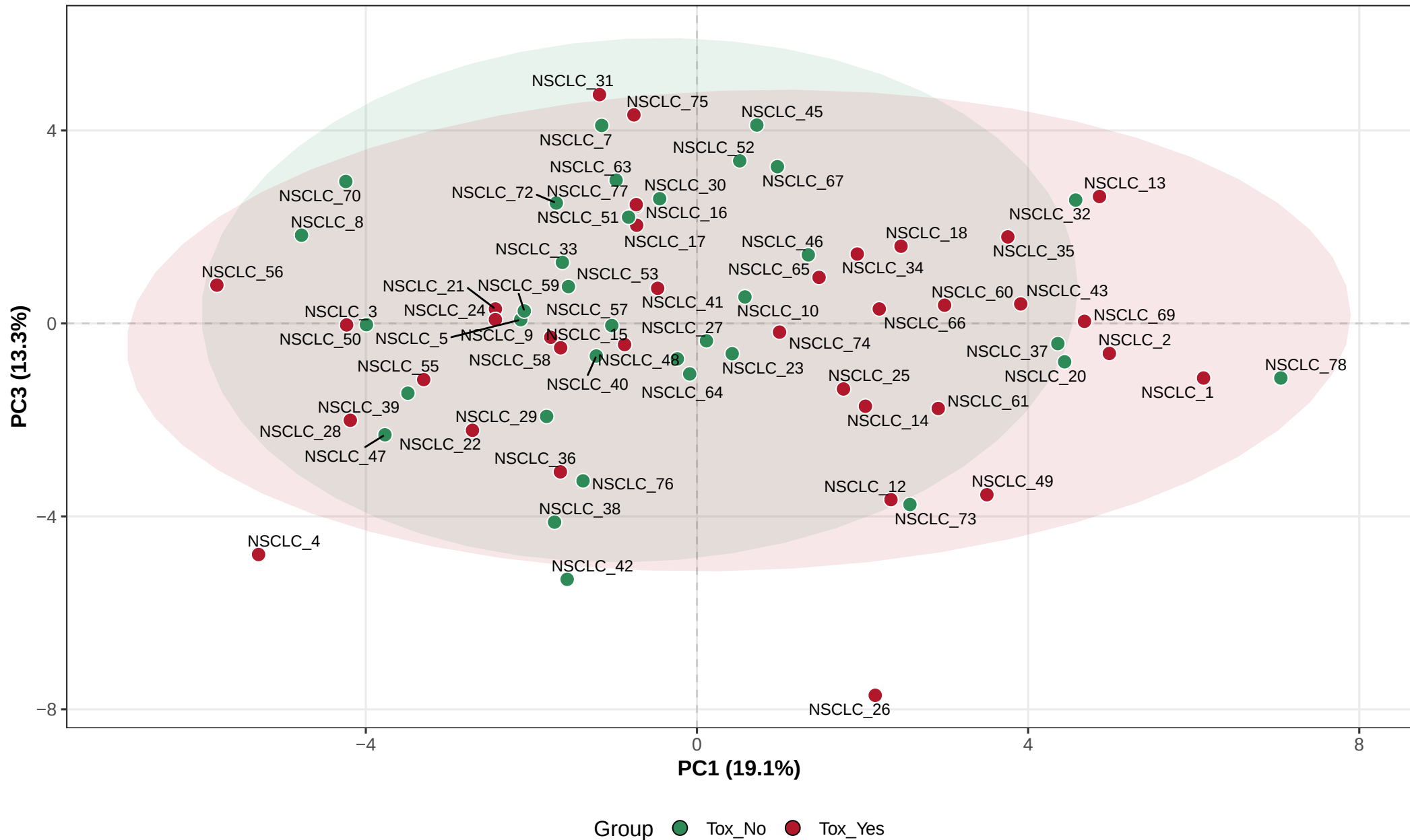
PCA (PC1 vs PC3)
