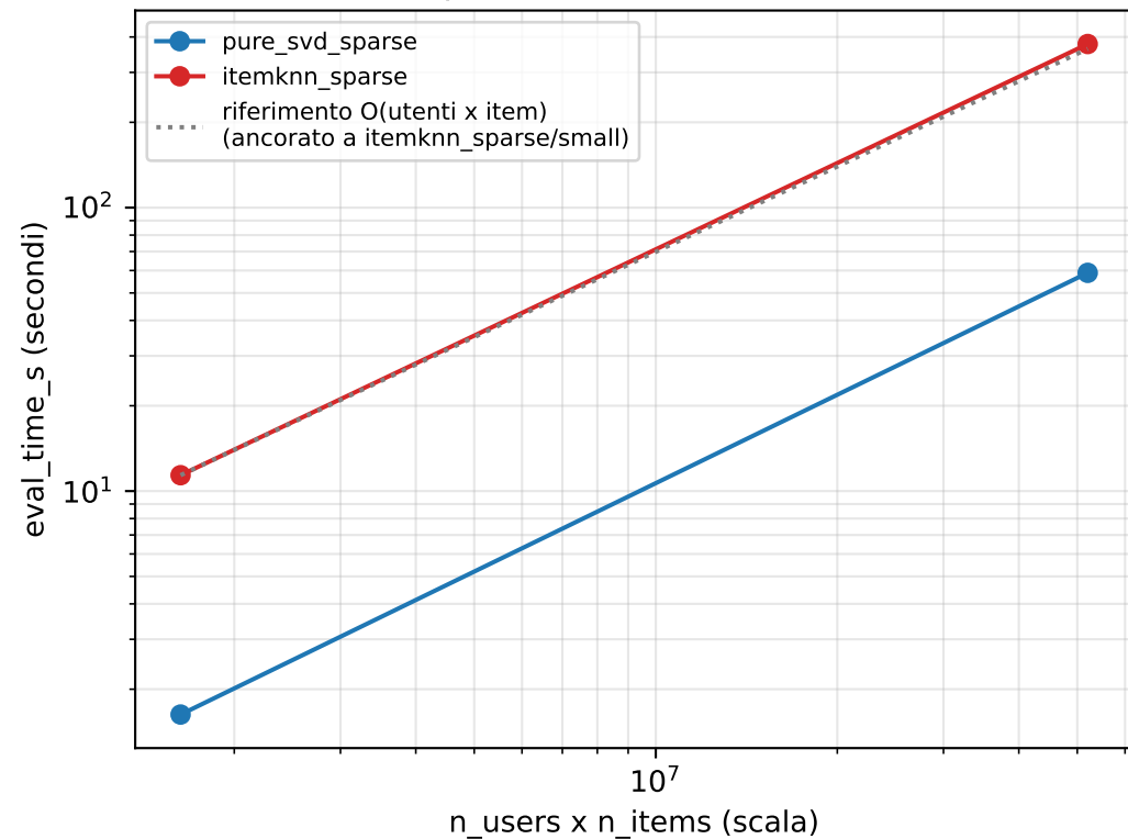
Tempo di valutazione vs scala
