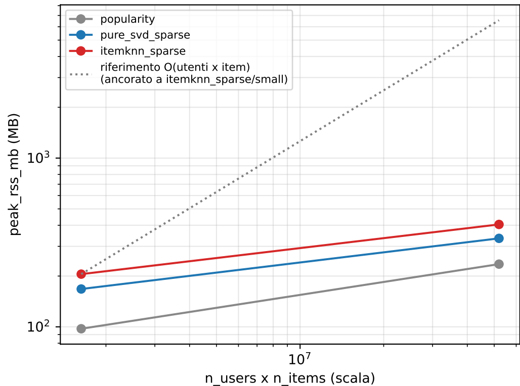
Picco di memoria vs scala
