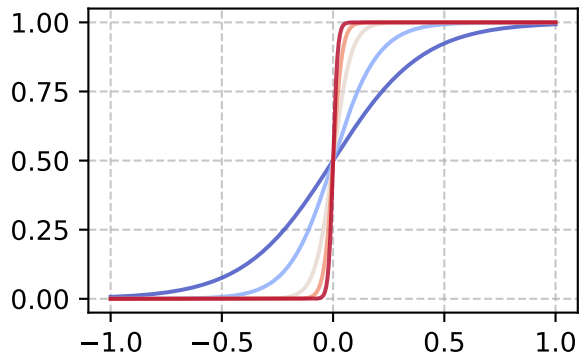
e^{c[x = 0]}
