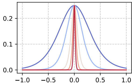
e^{c[x = 0]}
