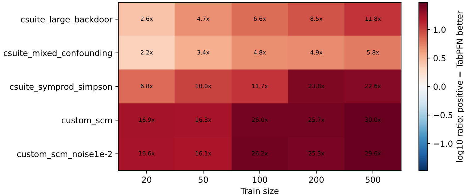
TabularARGN / TabPFN DAG-aware median loss ratio - CMD
