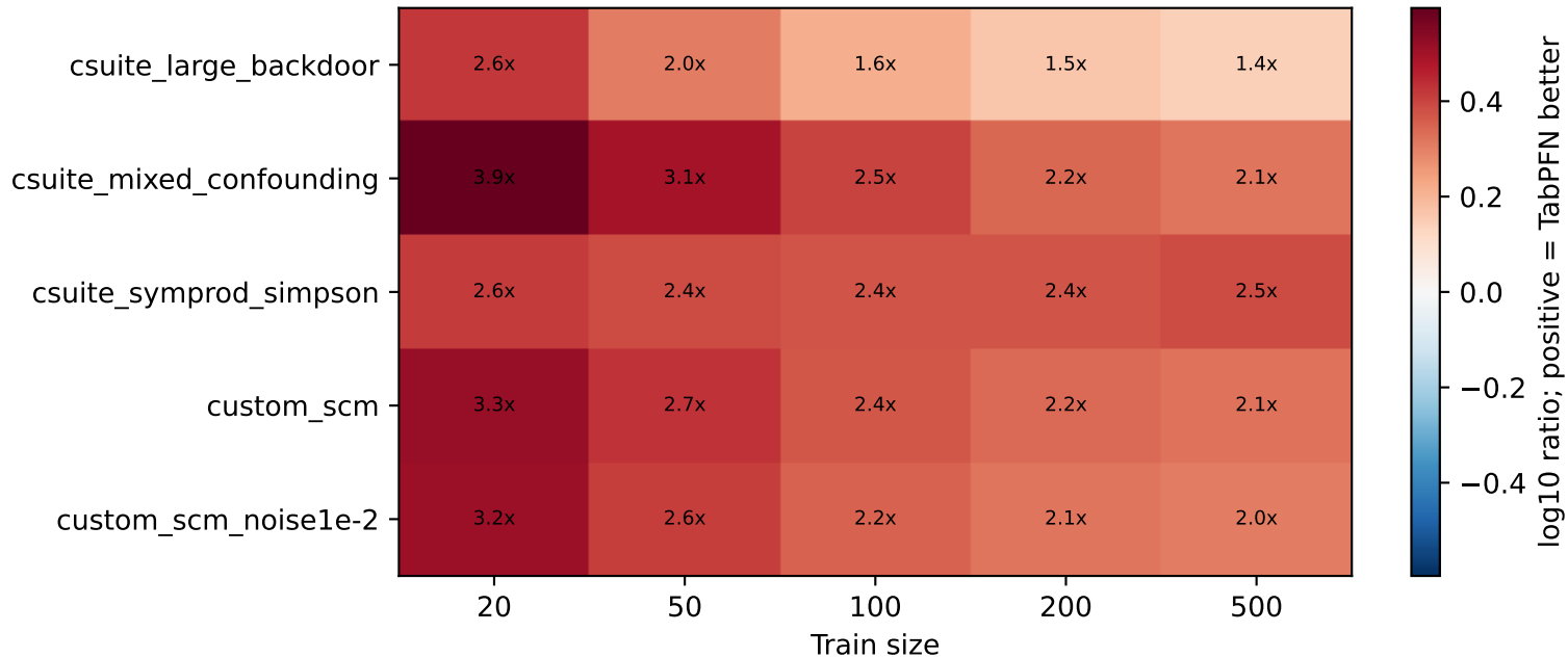
TabularARGN / TabPFN DAG-aware median loss ratio - kMTVD
