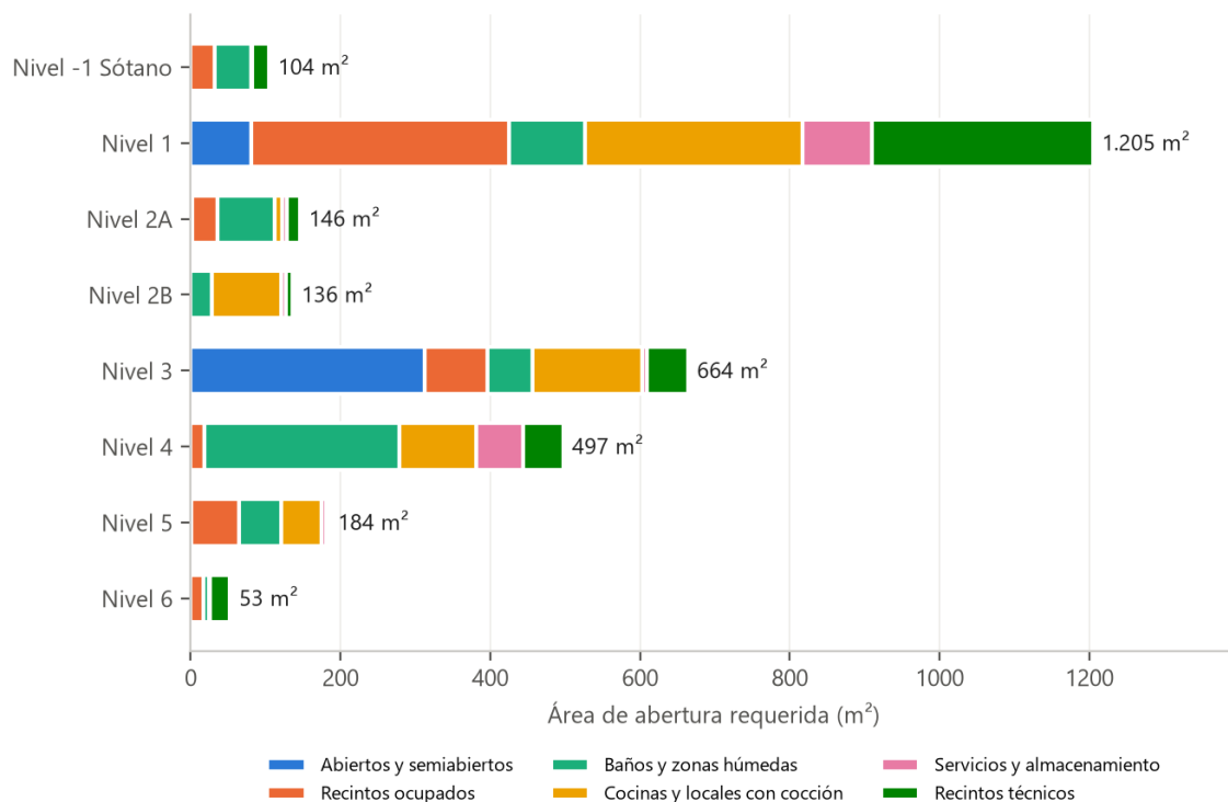
Ilustración 4 Área de abertura requerida por nivel y régimen de ventilación
