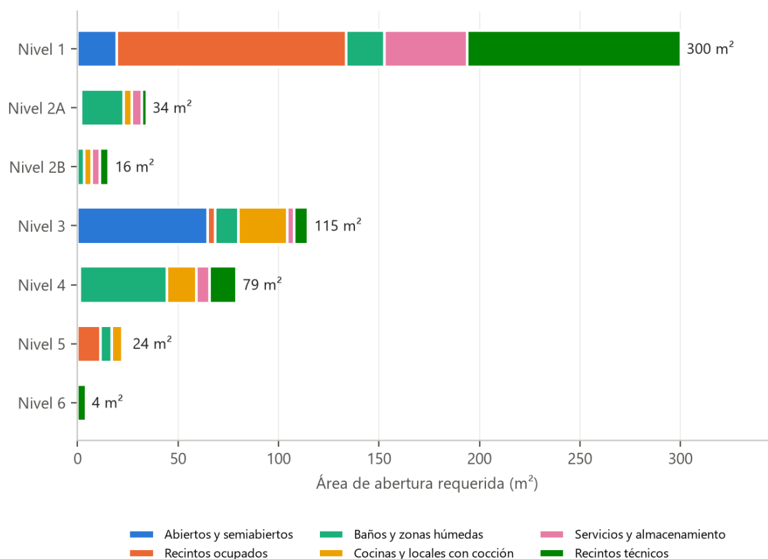
Ilustración 13 Tribuna Oriental – abertura requerida por nivel y régimen
