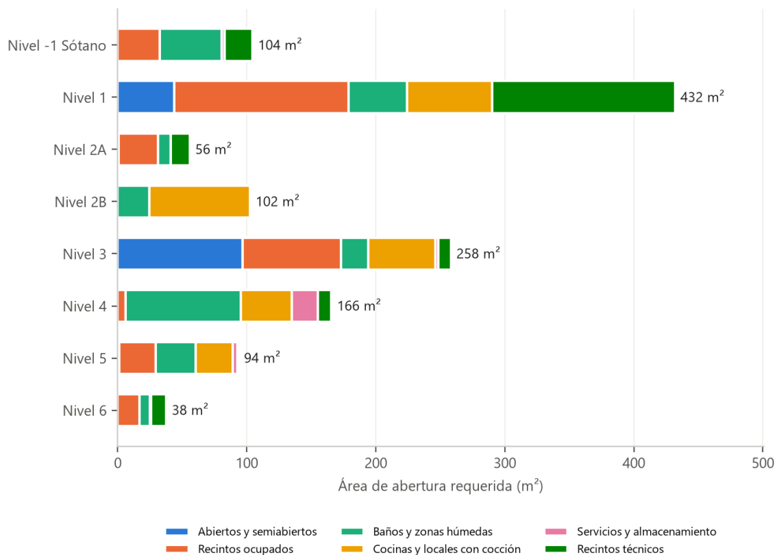
Ilustración 11 Tribuna Occidental – abertura requerida por nivel y régimen
