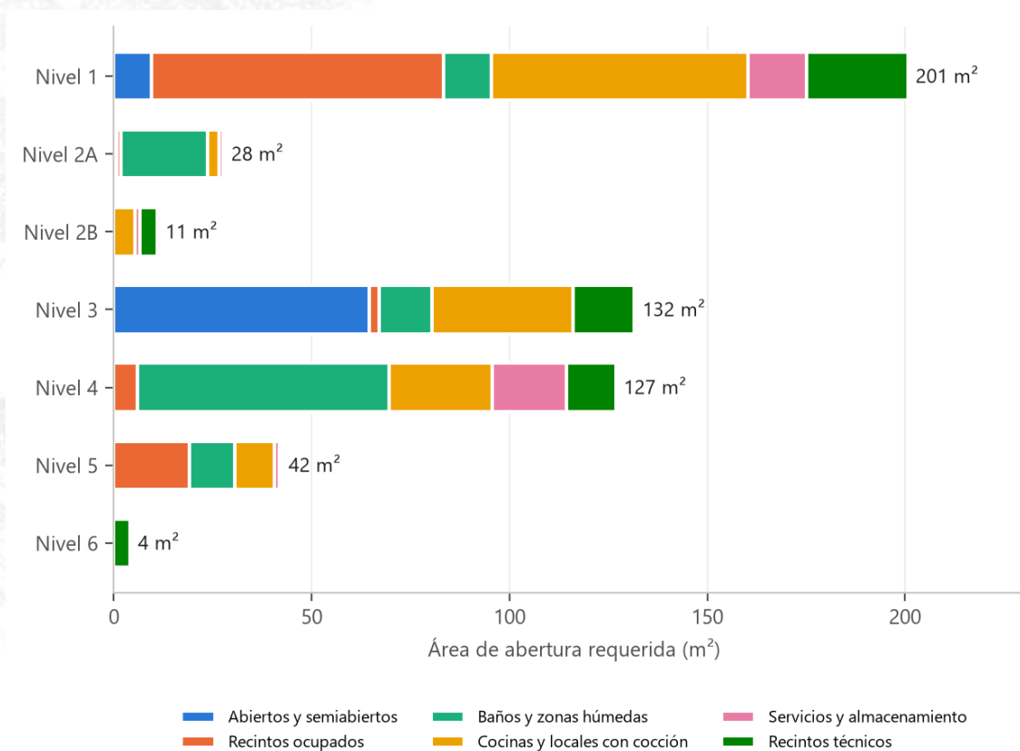
Ilustración 12 Tribuna Norte – abertura requerida por nivel y régimen
