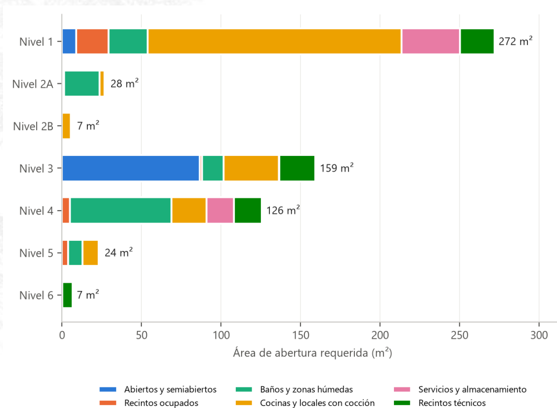
Ilustración 14 Tribuna Sur – abertura requerida por nivel y régimen
