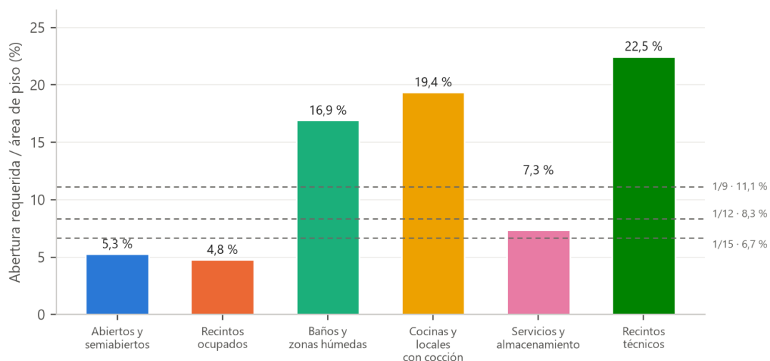
Ilustración 9 Índice de abertura requerida por régimen frente a las relaciones de referencia
