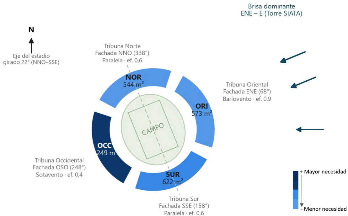
Área total de abertura requerida por tribuna (m 2 ) · planta esquemática con norte real arriba
