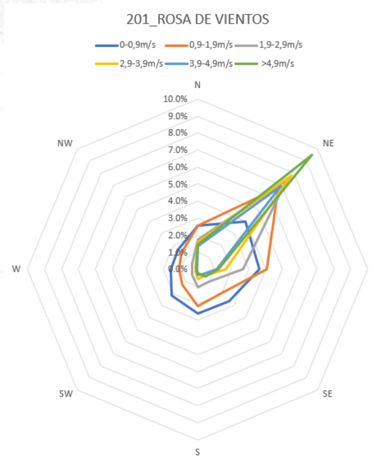
Ilustración 2. Rosa de vientos promedio histórico del lugar – SIATA 201
