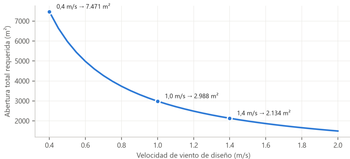
Ilustración 10 Sensibilidad del área total de abertura a la velocidad de viento de diseño
