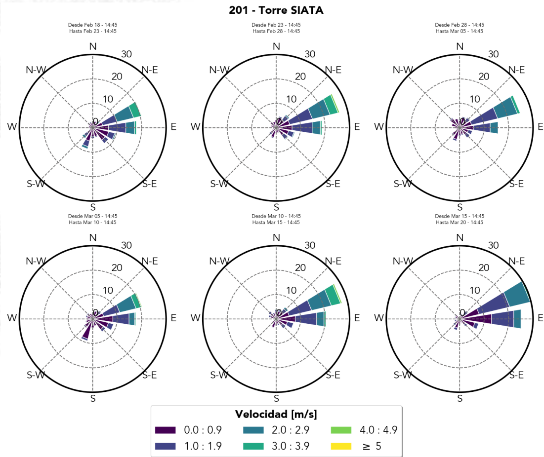
Ilustración 1 Rosa de vientos de la Torre SIATA (estación 201)
