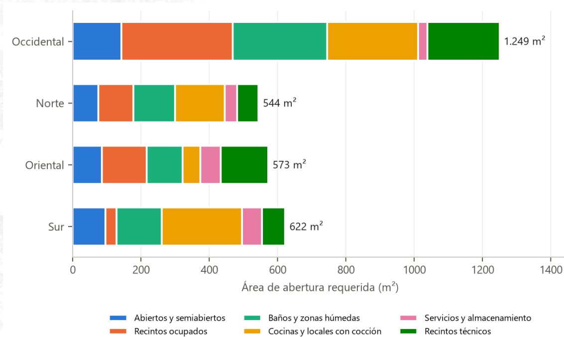
Ilustración 8 Área de abertura requerida por tribuna y régimen de ventilación
