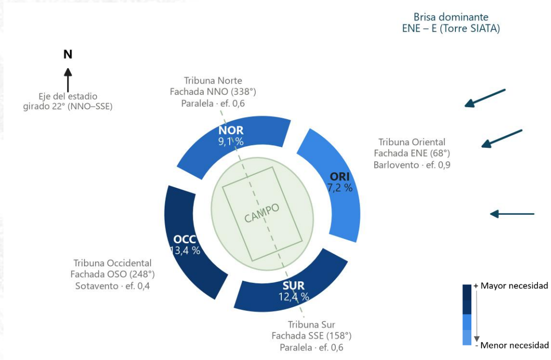
Ilustración 6 Esquema espacial – índice de abertura en recintos cerrados por tribuna
