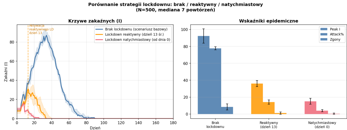
Rysunek 3: Porównanie strategii lockdownu: brak / reaktywny (aktywacja dzień \approx 13 , gdy I \geq 25 ) / natychmiastowy (od dnia 0). Opóźnienie 13 dni zwiększa attack rate 3,5-krotnie.
