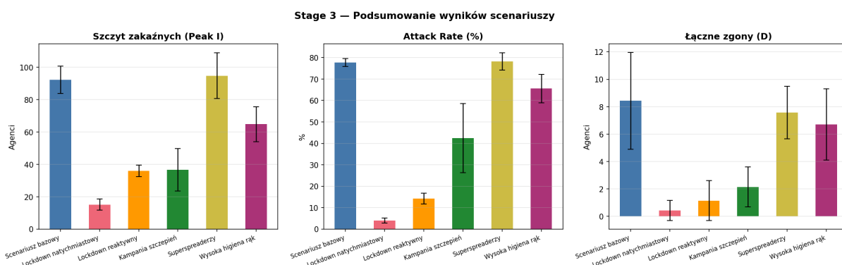
Rysunek 5: Porównanie kluczowych wskaźników: szczyt zakaźnych, attack rate i liczba zgonów dla sześciu scenariuszy. Słupki błędów: odchylenie standardowe między powtórzeniami.
