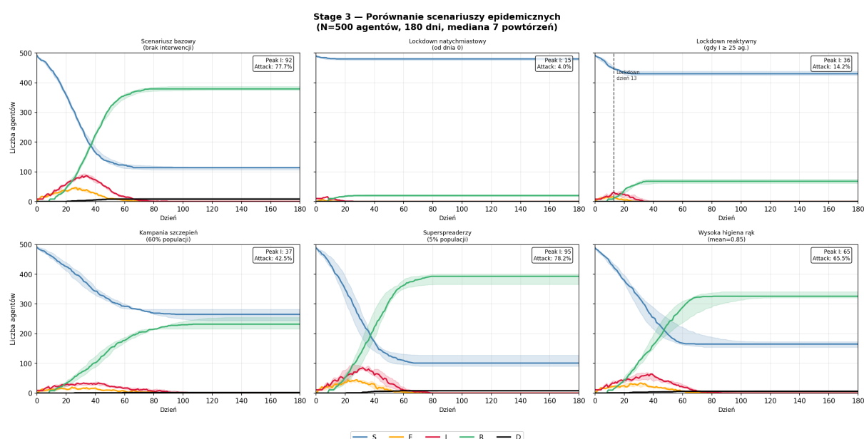
Rysunek 4: Krzywe SEIRD dla sześciu scenariuszy Stage 3 (siatka 2 \times 3 ). Linie ciągłe – mediana 7 powtórzeń; pasma – IQR. Pionowa przerywana w Sc. 2b oznacza moment aktywacji lockdownu.
