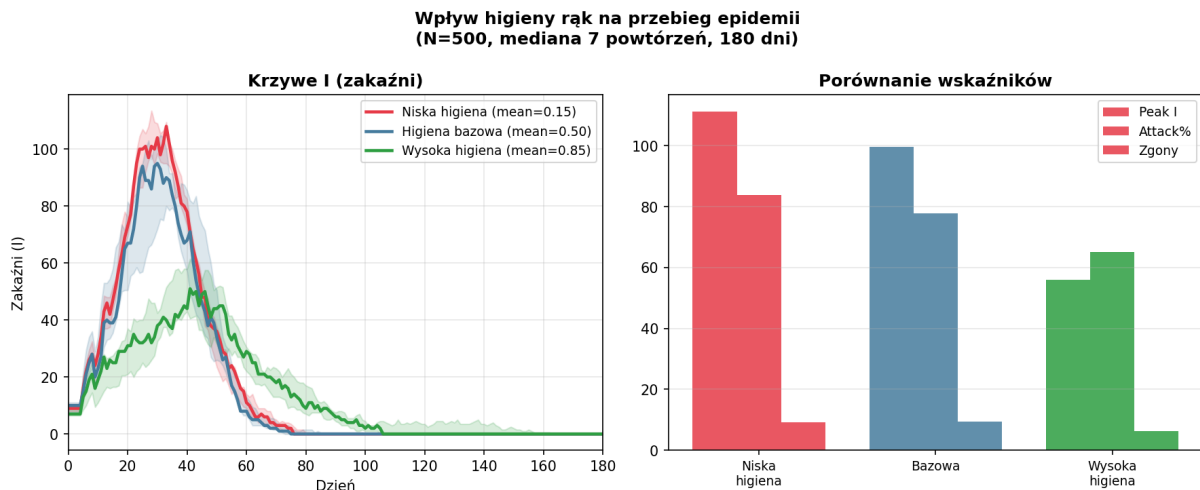
Rysunek 6: Wpływ poziomu higieny rąk ( \Theta_H ) na przebieg epidemii: krzywe zakaźnych (lewo) i porównanie wskaźników (prawo) dla trzech populacji.
