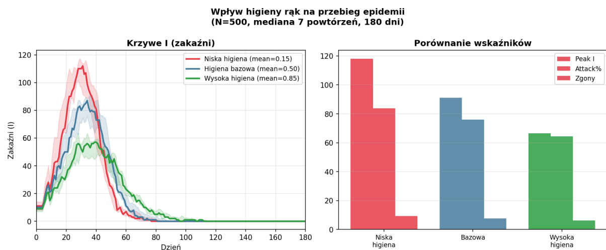
Rysunek 7: Wpływ poziomu higieny rąk ( \Theta_H ) na przebieg epidemii: krzywe zakaźnych (lewo) i porównanie wskaźników (pravo) dla trzech populacji.
