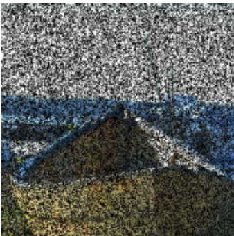
WL^{1,2}(B)
