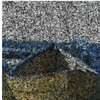
WL^{1,2}(C)
