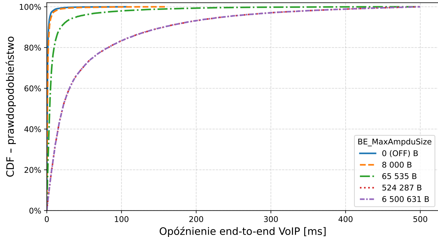
Scenariusz 1: wpływ limitu A-MPDU na CDF opóźnień VoIP Wi-Fi 6 (802.11ax), 5 stacji tła, 10 powtórzeń (pooled)
