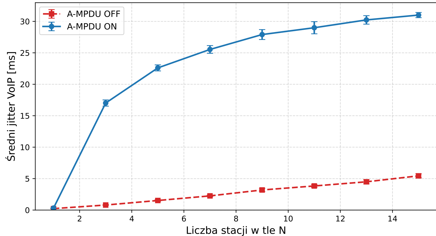
Scenariusz 2: średni jitter VoIP vs liczba stacji tła Wi-Fi 6 (802.11ax), 10 powtórzeń, 95% CI
