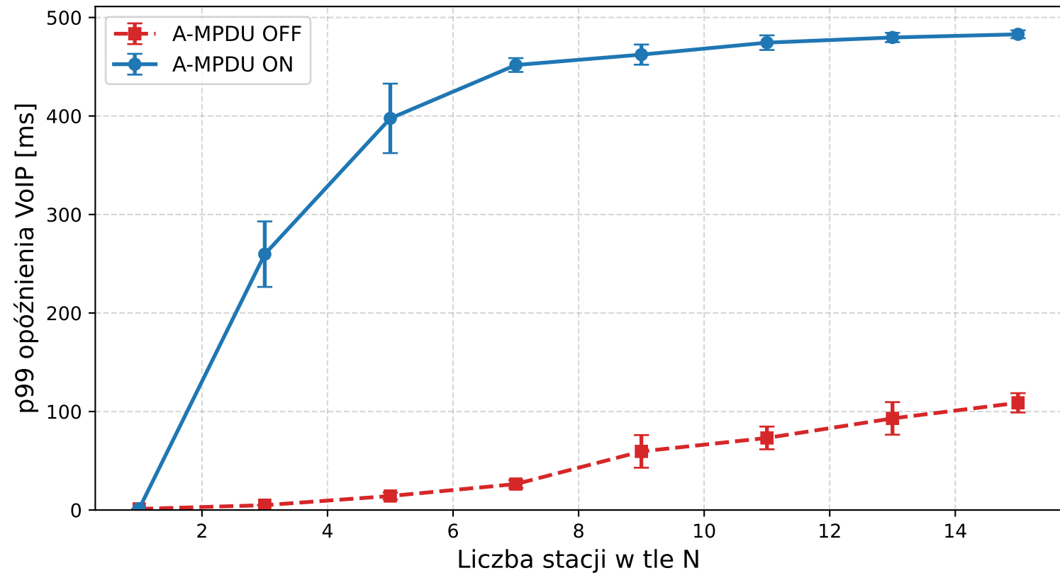
Scenariusz 2: p99 opóźnień VoIP vs liczba stacji tła Wi-Fi 6 (802.11ax), 10 powtórzeń, 95% CI
