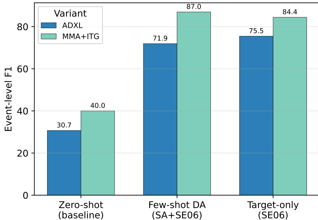
Event-level F1
