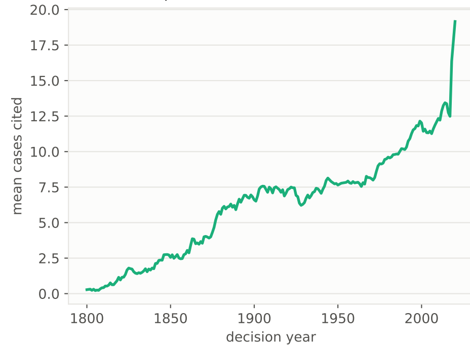
References per case
