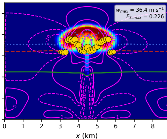
(c) WARM ( q_v fixa; RH variavel) + DYN_PLUS (d) WARM (RH fixa) + DYN_PLUS t \approx 20 min
