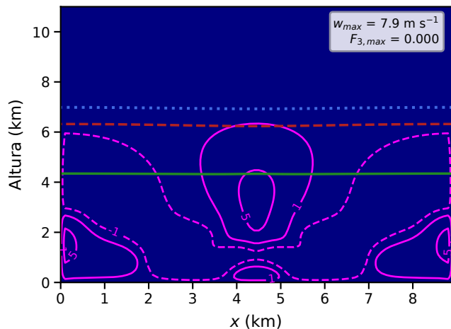
(c) WARM ( q_v fixa; RH variavel) + DYN_PLUS (d) WARM (RH fixa) + DYN_PLUS t \approx 20 min
