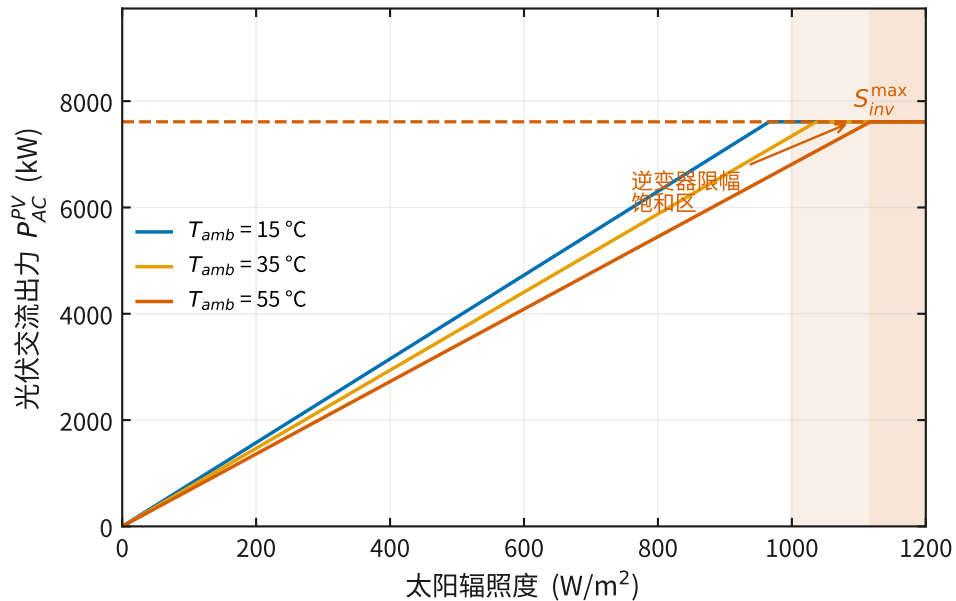
光伏逆变器截断与功率包络
