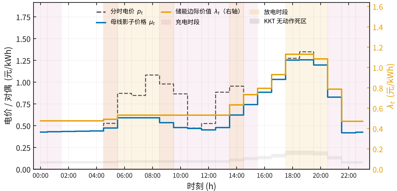
KKT 对偶影子价格与储能边际价值
