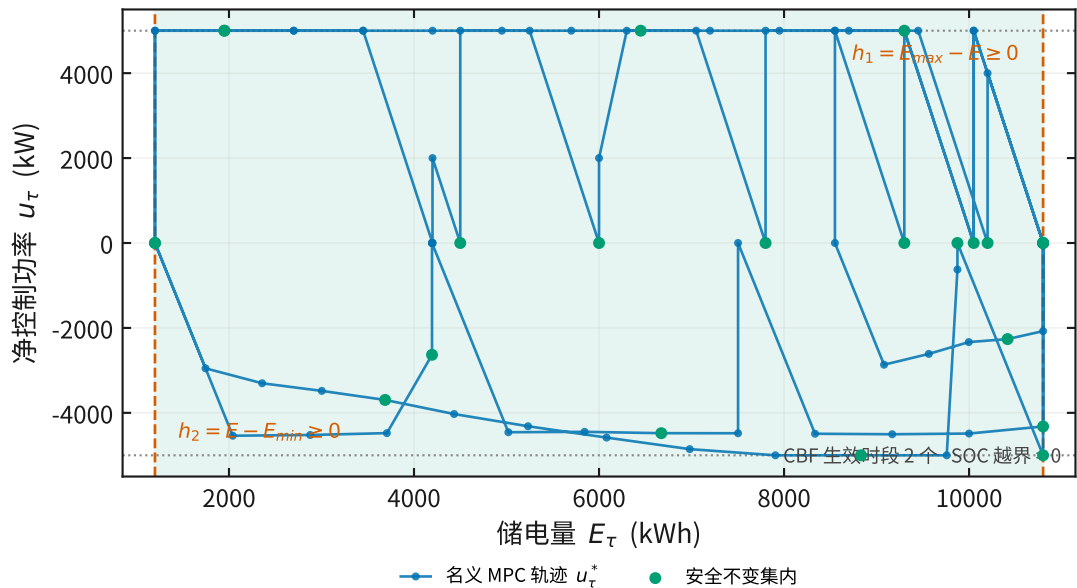
CBF 相空间安全过滤
