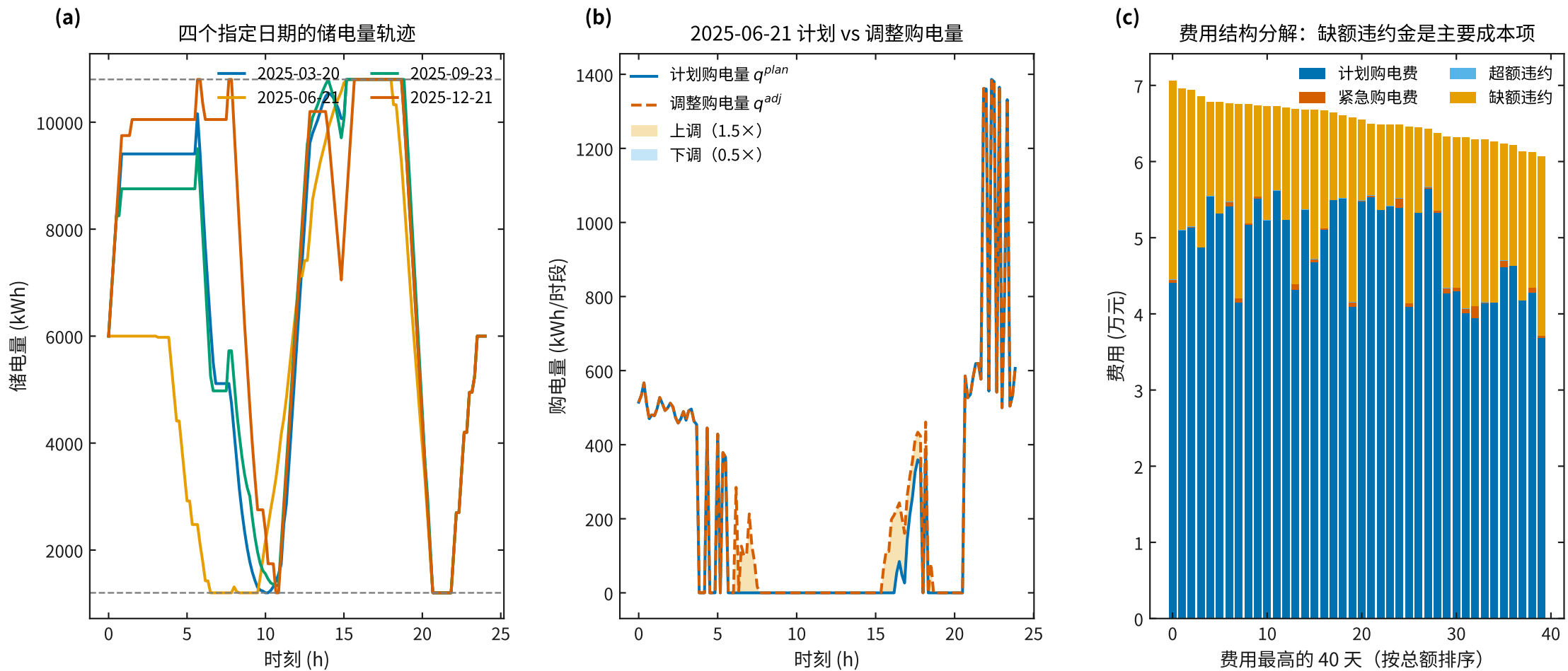
图7 问题3：储电量轨迹、计划/调整购电量与结算费用结构
