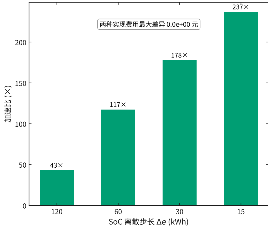
(b) 加速比（状态数越大收益越高）
