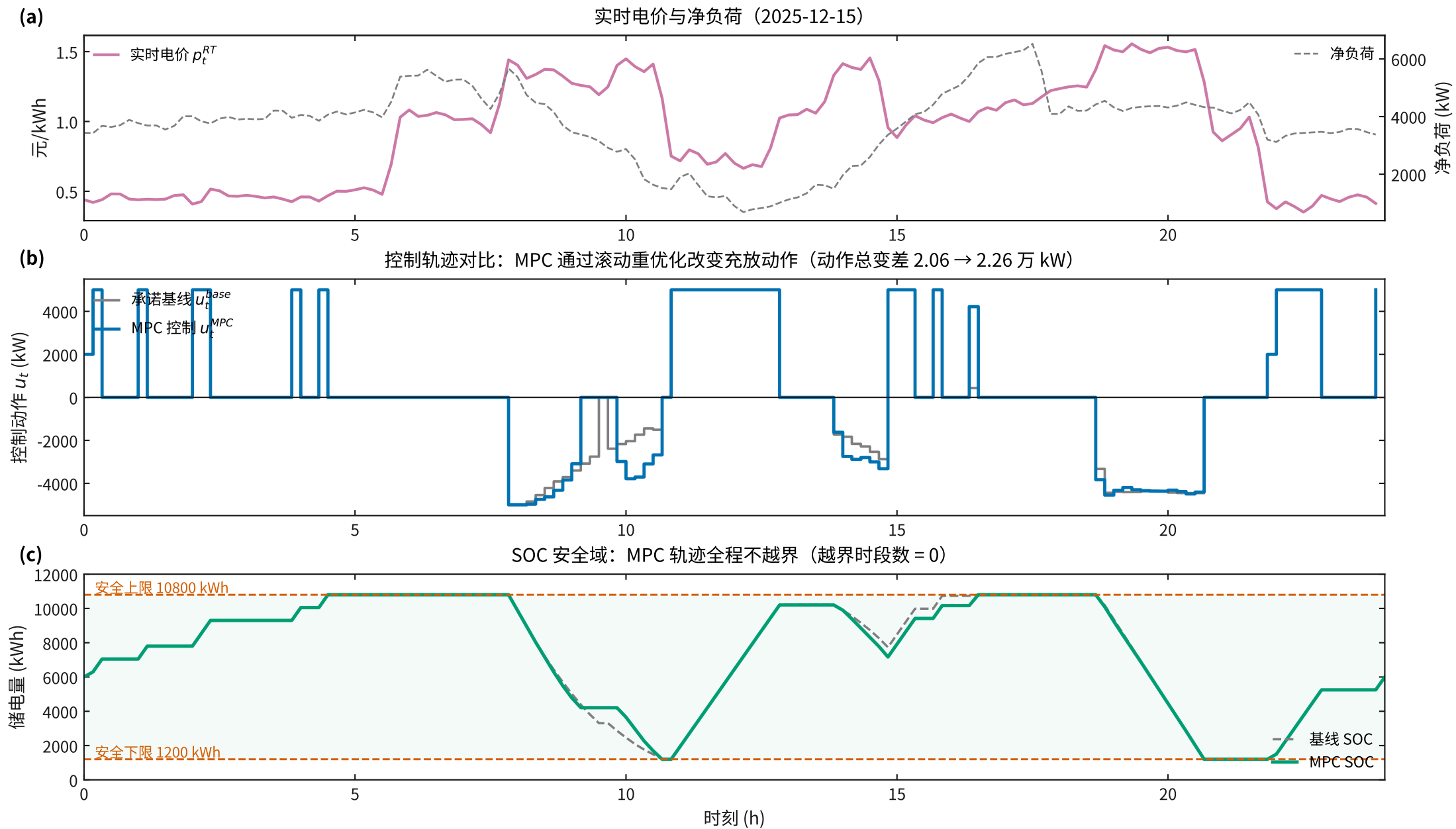
Fig.7 Q4 实时控制轨迹与 SOC 安全域
