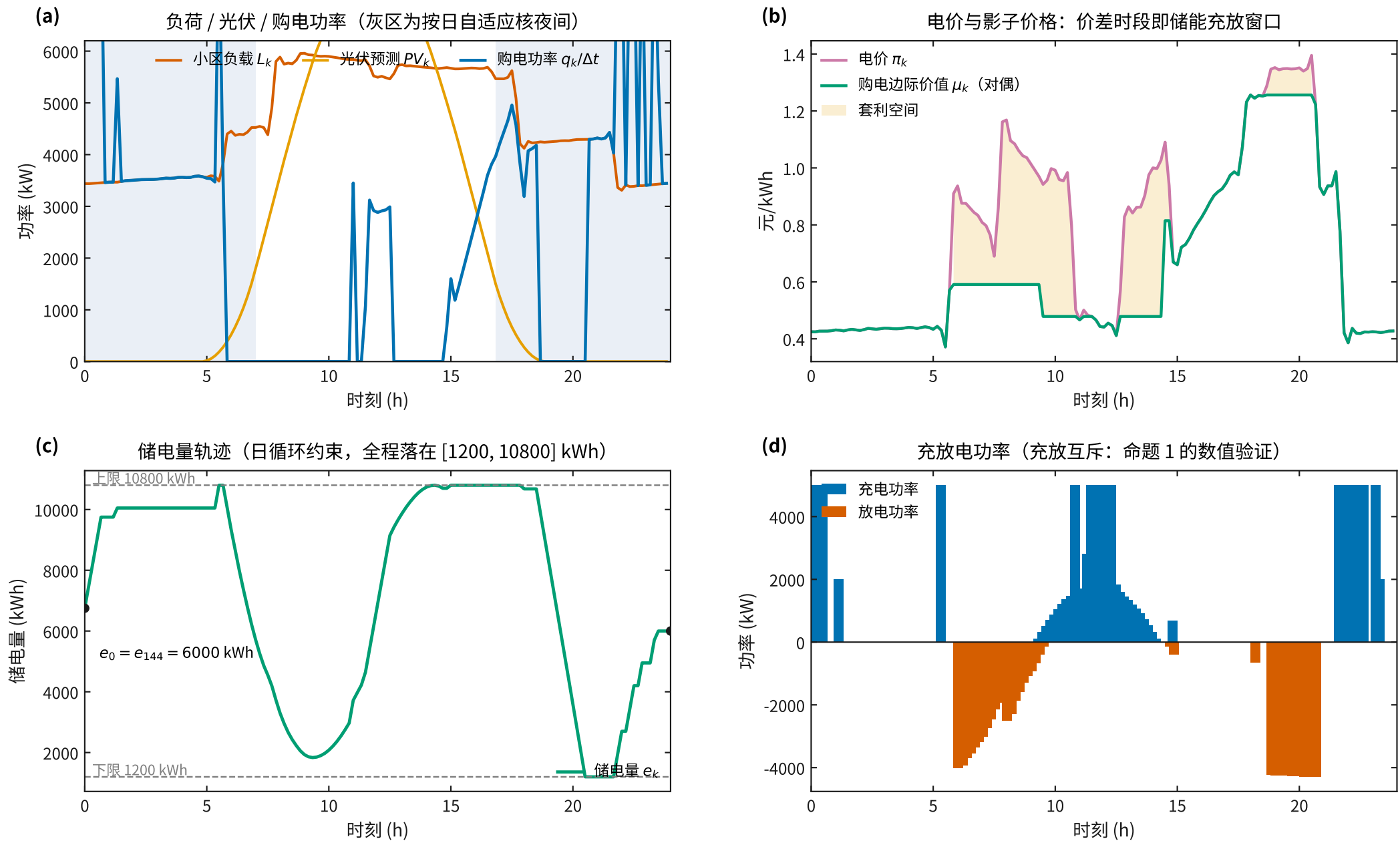
图1 问题1 代表性日最优计划：全天 35126.95 元，较 B2 基线 48052.05 元下降 26.90%
