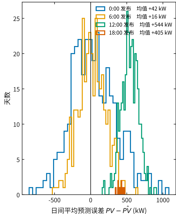
(c) 四时次预报误差分布 (偏差诊断)
