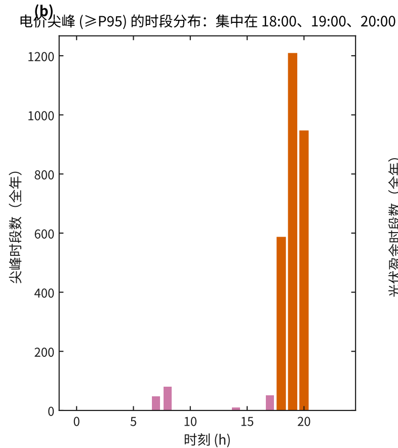
Fig.D5 爬坡与极值特征：波动强度、价格尖峰与光伏盈余
