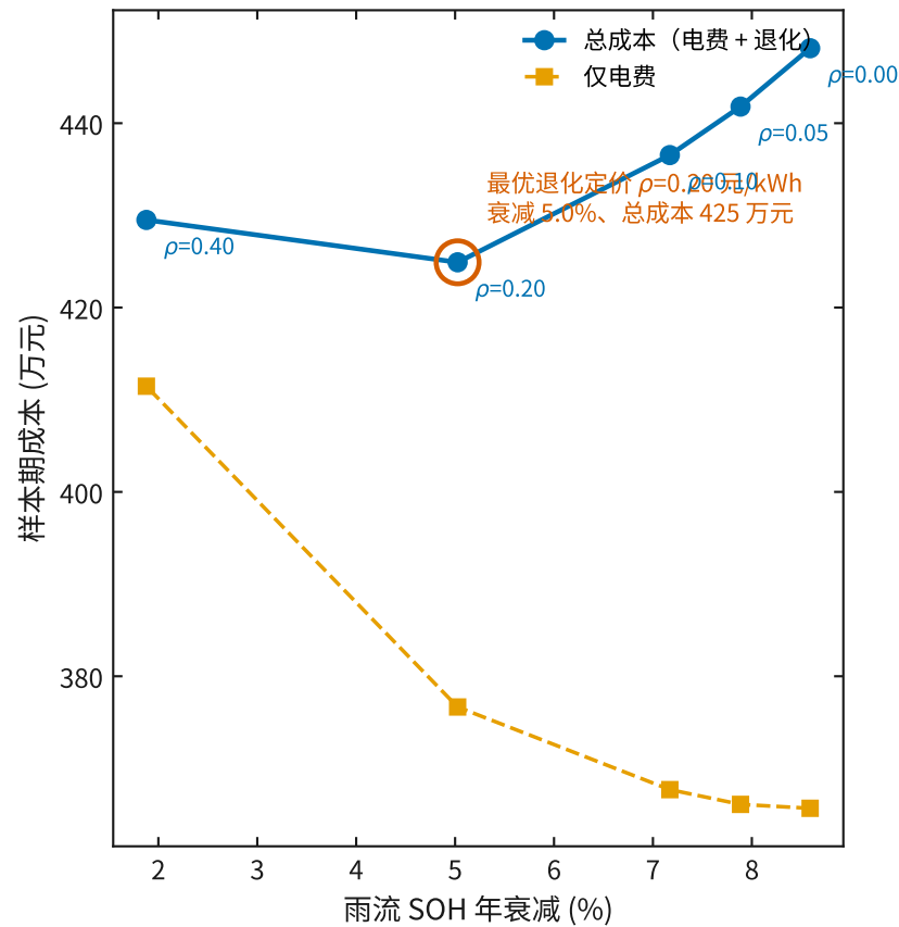
(b) 退化定价前沿：忽略退化并非经济最优
