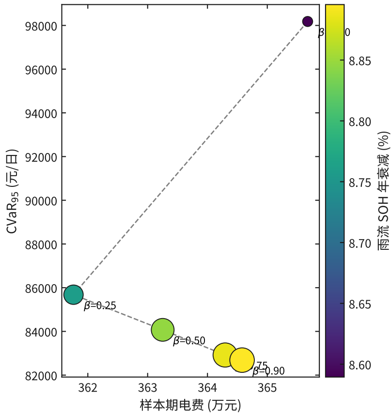
(a) 风险层 Pareto (气泡/颜色 = 真实 SOH 衰减)
