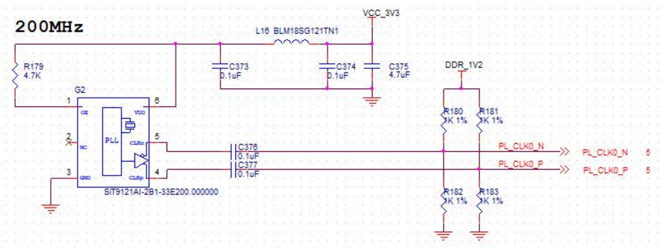
图 6-4 PL系统时钟源
