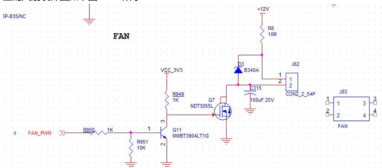
图 28-1 开发板原理图中风扇设计
