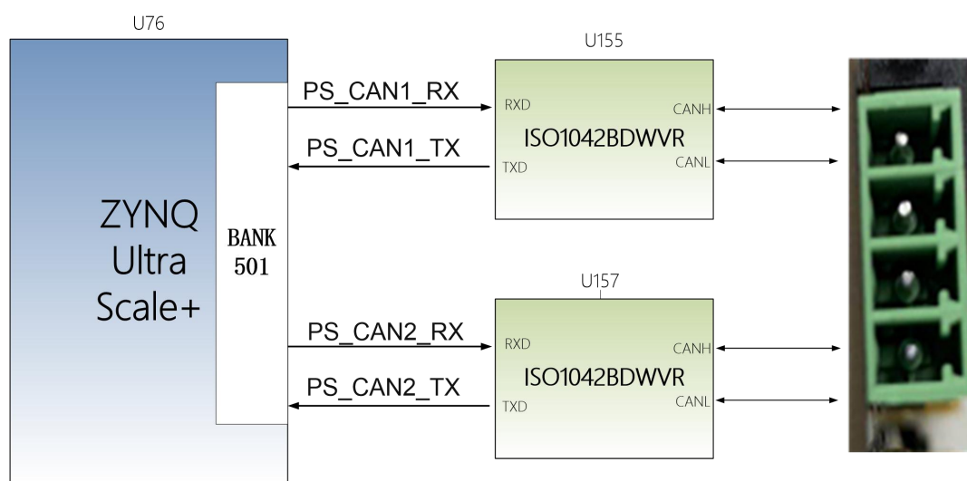
图 15-1 PS 端 CAN 收发芯片的连接示意图
