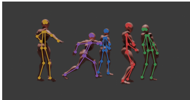
K=5
