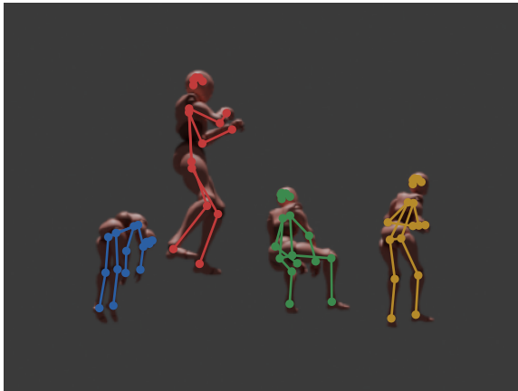
K=4
