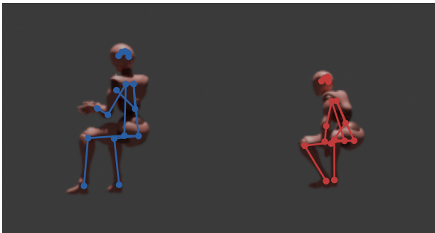
K=2
