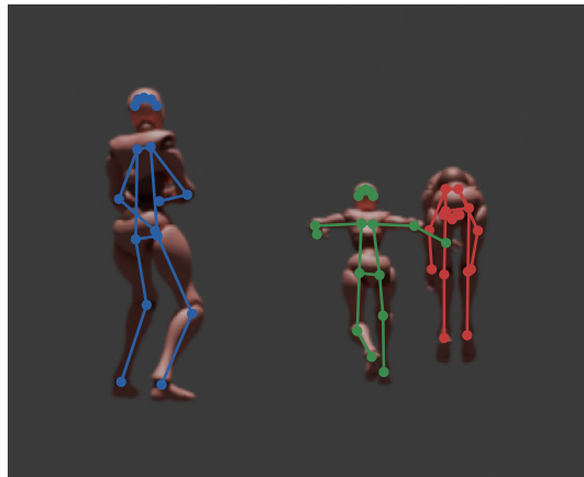
K=3
