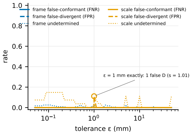
(d) decision rates vs. tolerance (exact truth)
