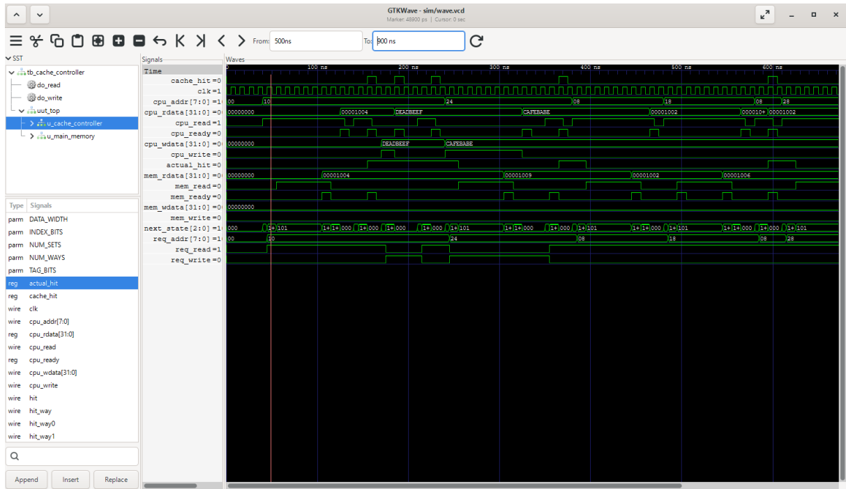
Figure 3: Validação da política de substituição LRU. Os endereços 8'h08, 8'h18 e 8'h28 mapeiam para o mesmo conjunto da cache. Após o novo acesso a 8'h08, esse bloco se torna o mais recentemente usado. Assim, quando 8'h28 é carregado, o bloco correspondente a 8'h18 é substituído.
