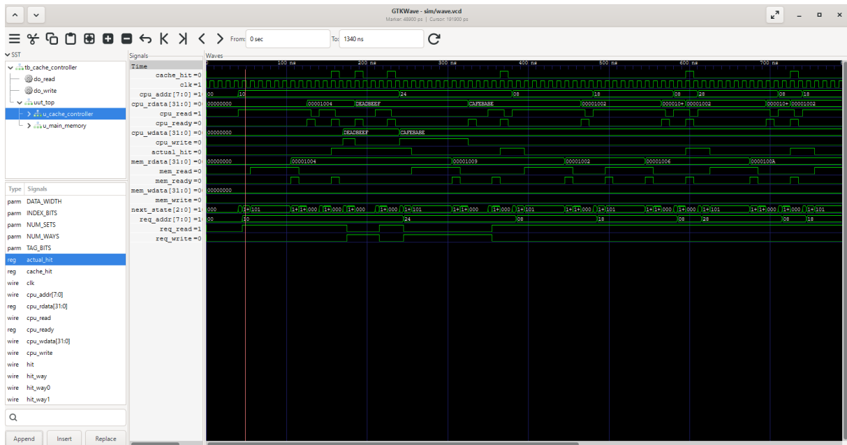
Figure 1: Visão geral da simulação do controlador de cache, mostrando operações de leitura, escrita, misses, hits, substituição LRU e write-back.
