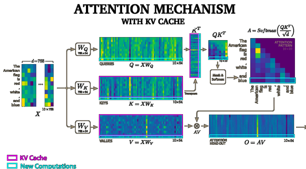
Figure 2: Интуитивна схема на attention механизма
