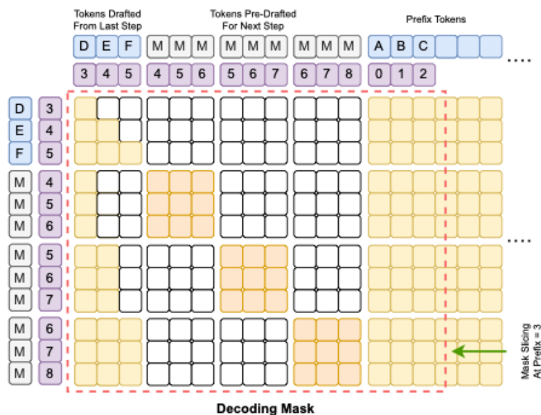
Figure 14: Структурирана маска за TiDAR decode/преддрафт логика (diagram from TiDAR paper)
