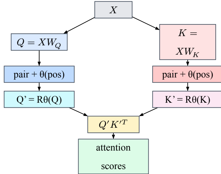
Figure 6: RoPE: позиционно-зависима ротация в Q/K преди attention score
