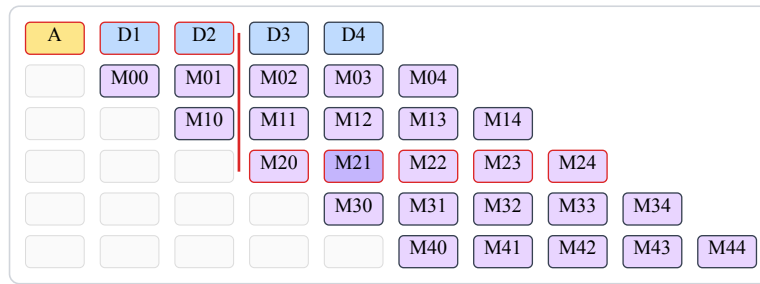
Figure 18: Триъгълна визуализация на verify/predraft зависимостите; пример с маркиран M21 При token M21:
