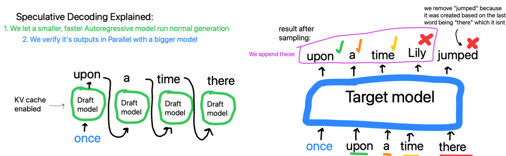
Figure 12: Базов speculative decoding (референтен случай)
