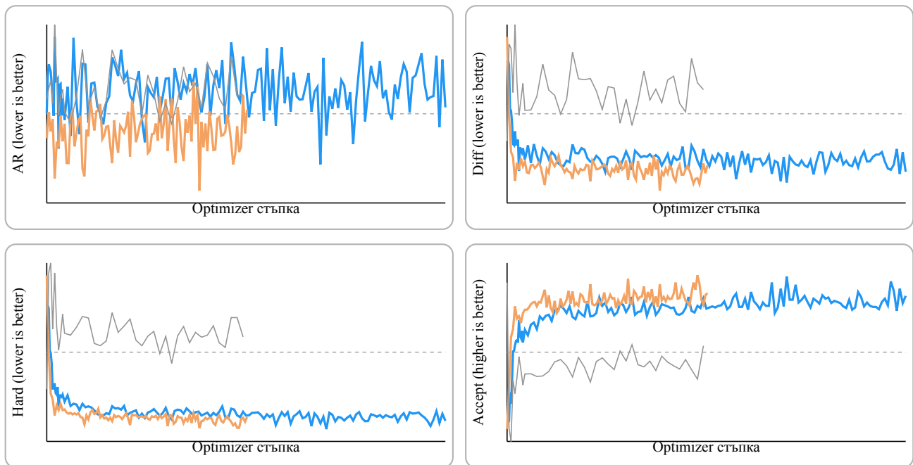
Figure 26: Обучителни метрики: 135М срещу 360М
