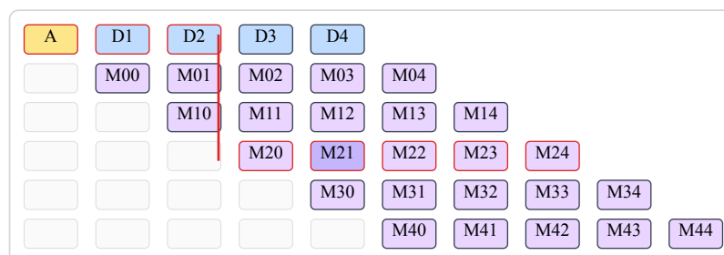
Figure 18: Триъгълна визуализация на verify/predraft зависимостите; пример с маркиран M_{21}
