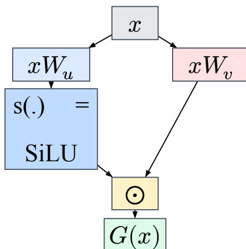
Figure 5: SwiGLU: два линейни пътя + gate + точково умножение
