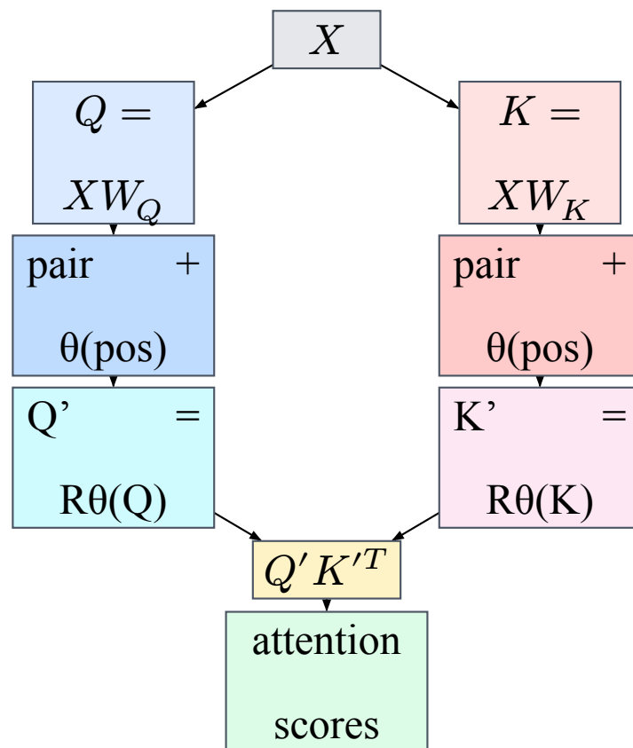
Figure 6: RoPE: позиционно-зависима ротация в Q/K преди attention score
