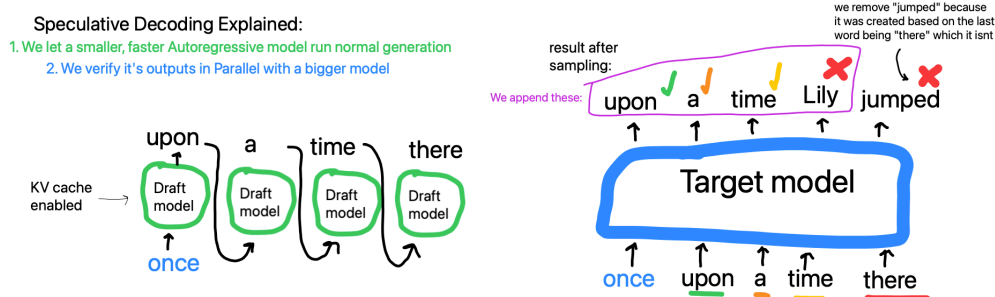
Figure 10: Базов speculative decoding (референтен случай за сравнение)
