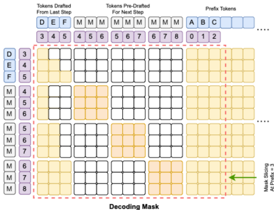
Figure 5: Маска за TiDAR decode/преддрафт логика
