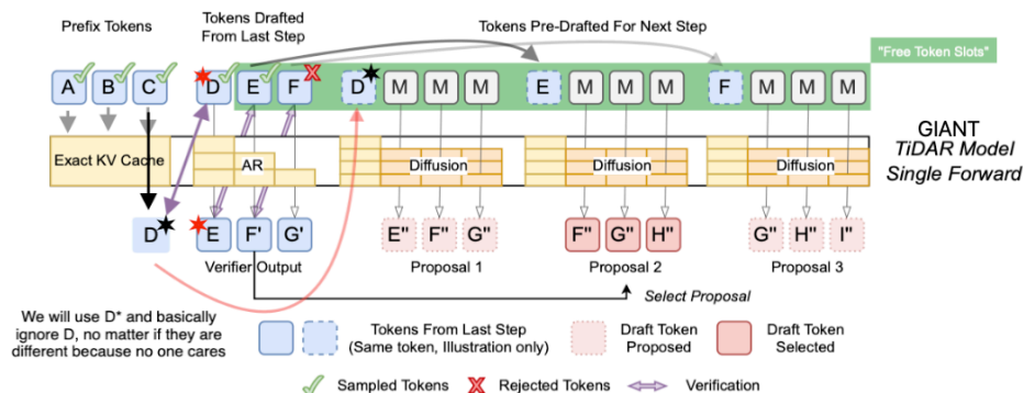
Figure 7: Иллюстрация на Anchor-TiDAR single-forward decode стъпка
