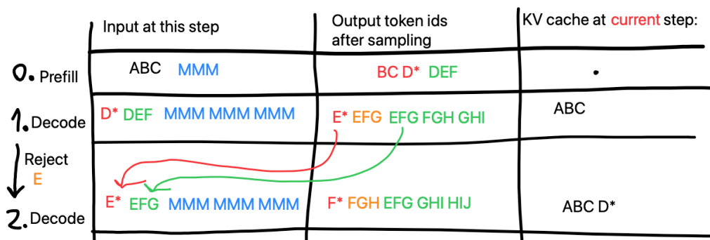
Figure 6: KV cache развитие по итерации при Anchor-TiDAR
