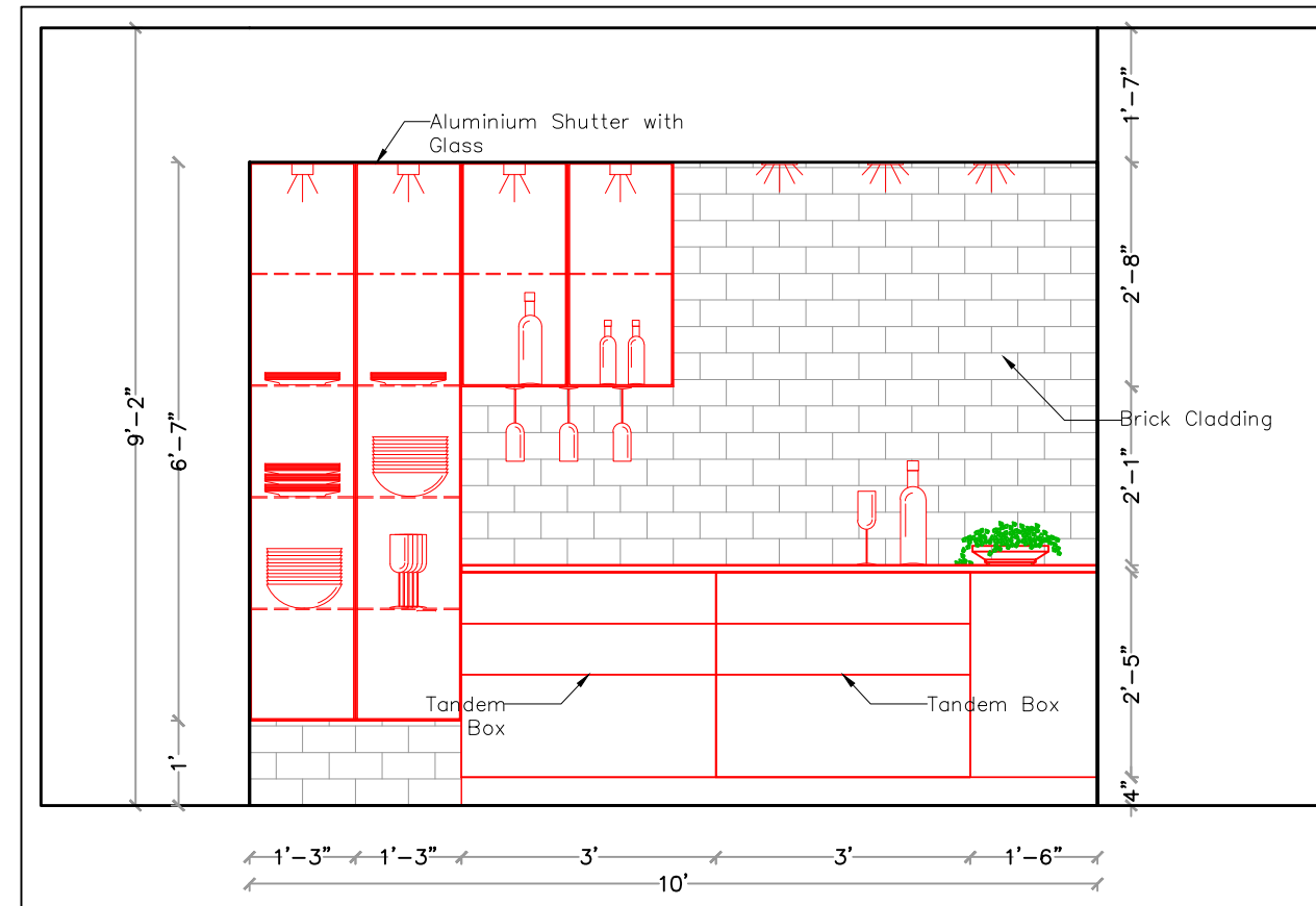
Elevation
