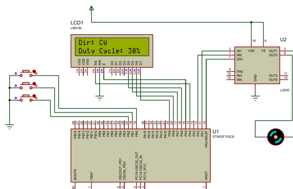
(ت) تنظیم دیوتی سایکل روی ۳۰ درصد
