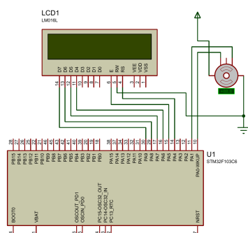
(ب) شماتیک کلی اتصالات انکودر و نمایشگر
