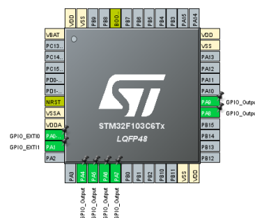
(ت) تنظیمات پایه‌های وقفه در STM32CubeIDE
