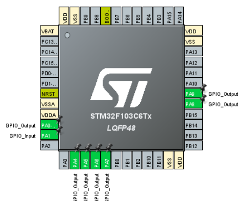
(آ) تنظیمات پایه‌ها در نرم‌افزار
